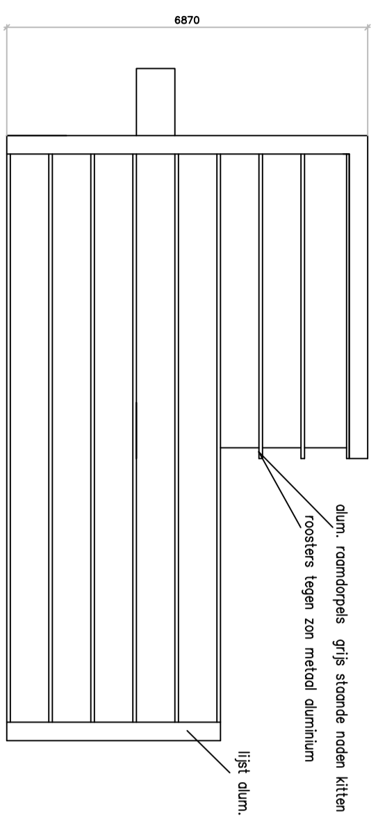
westgevel
